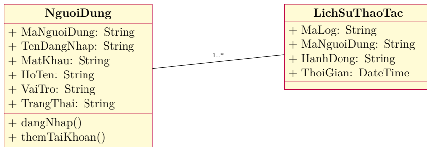
Figure 1: Class trong UC03 – Thêm tài khoản
